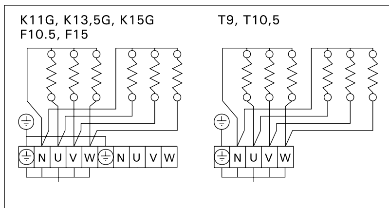
Rys. 5. Przylączy elektryczne pieca Obrázek 5. Zapojení topného tělesa
